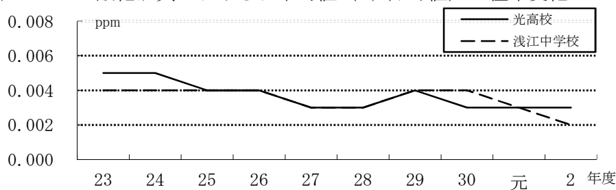
図－3 二酸化硫黄における日平均値（2％除外値）の経年変化
