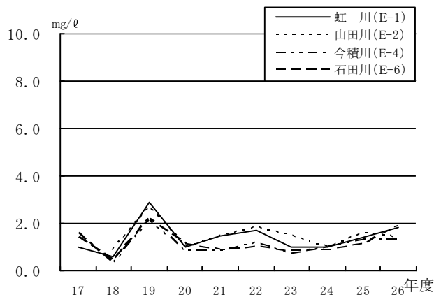
図-14 中小河川におけるBOD経年変化（年度平均値）
