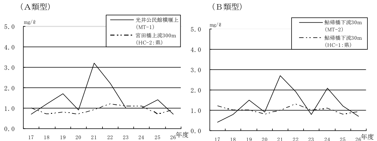
図-10 光井川水系における BOD 経年変化（年度平均値）
