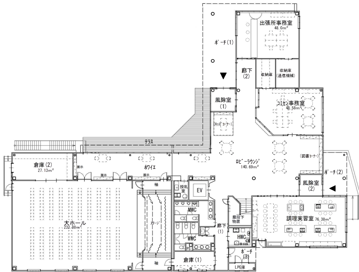
1階平面図
