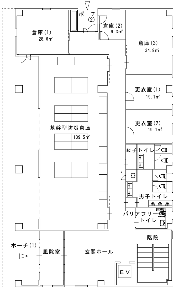
1階平面図
