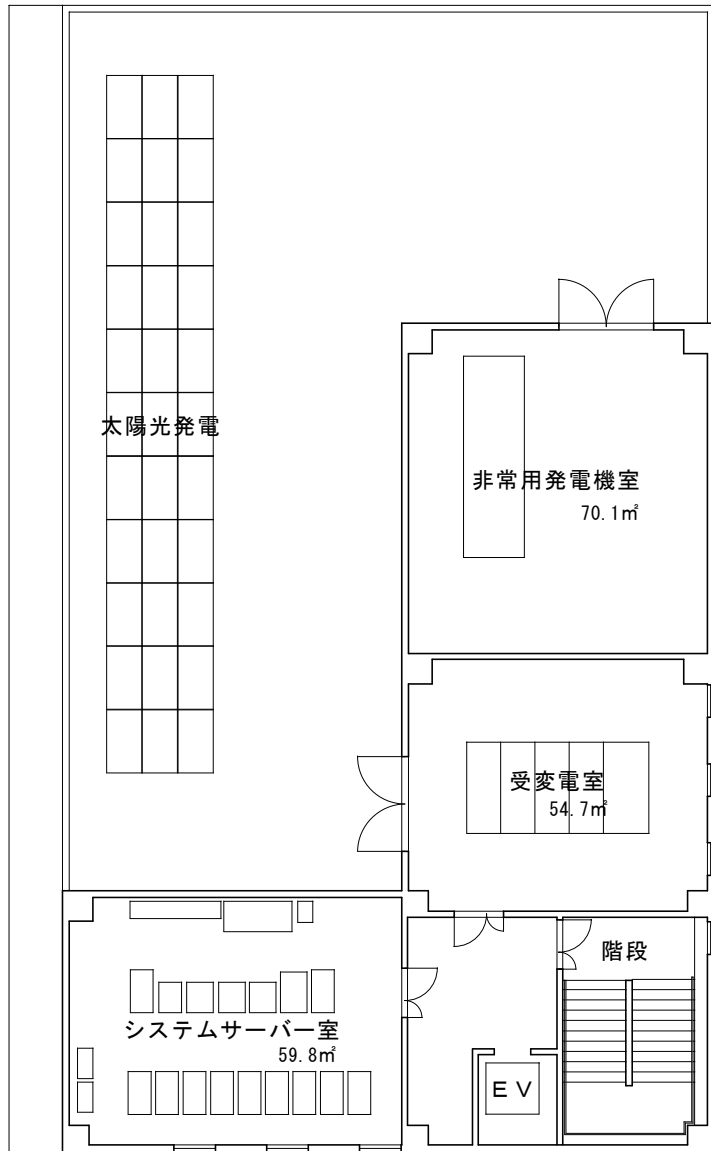
3階平面図
